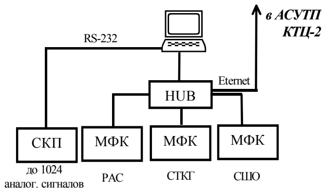
Рис. 4. АСУТП энергоблока №8 ТЭЦ-21 в 2001г.
